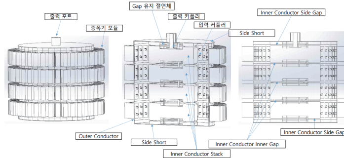
적층형 동축 공동 고주파 무선전력 결합장치 실시예 (1) ▲
