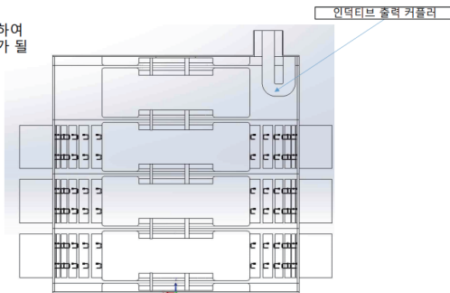
적층형 동축 공동 고주파 무선전력 결합장치 실시예 (2) ▲
